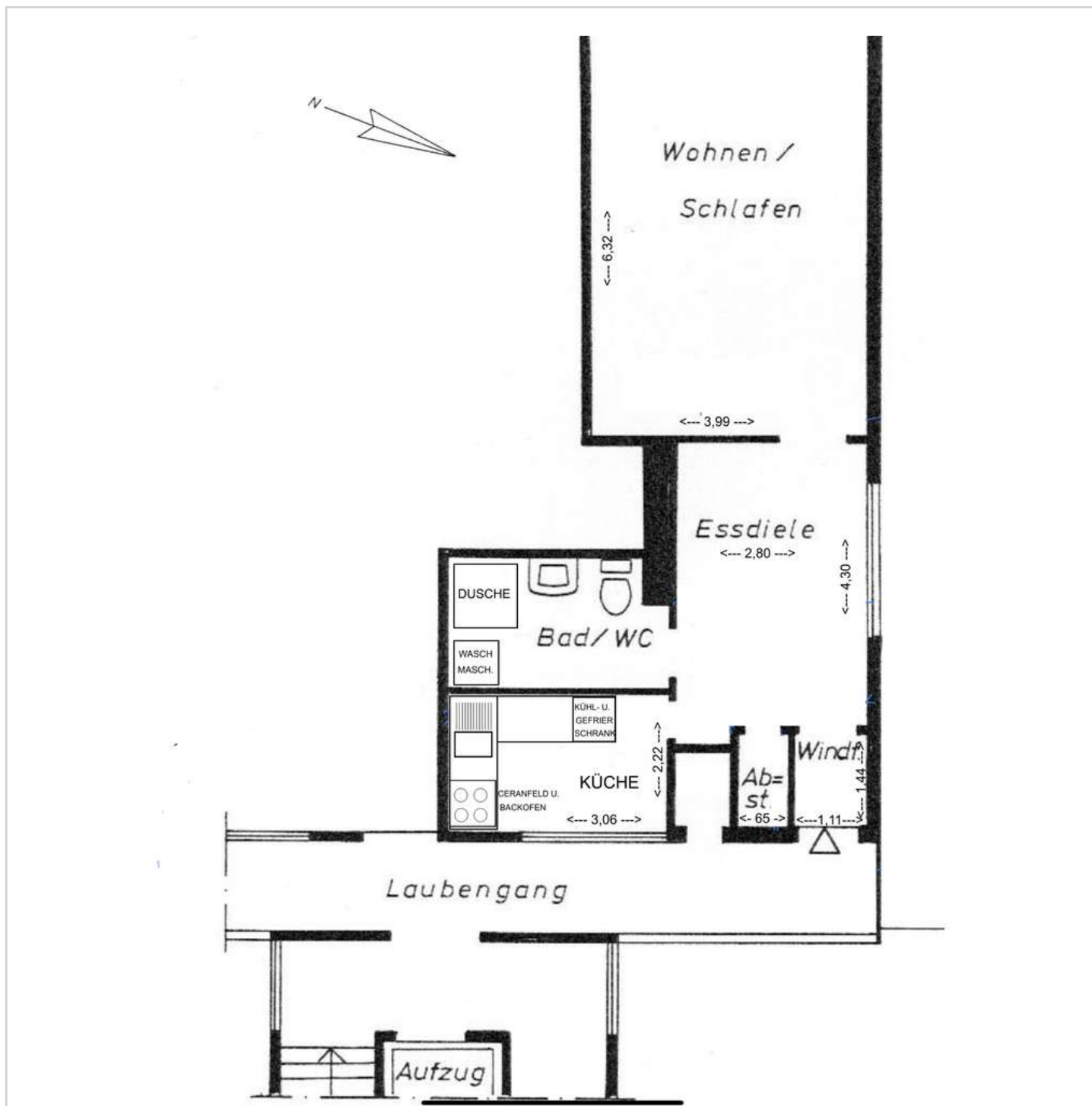
Grundriss 2022
