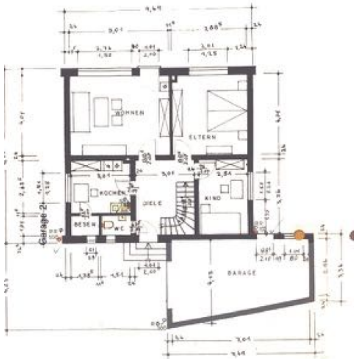
ERDGESCHOSS
