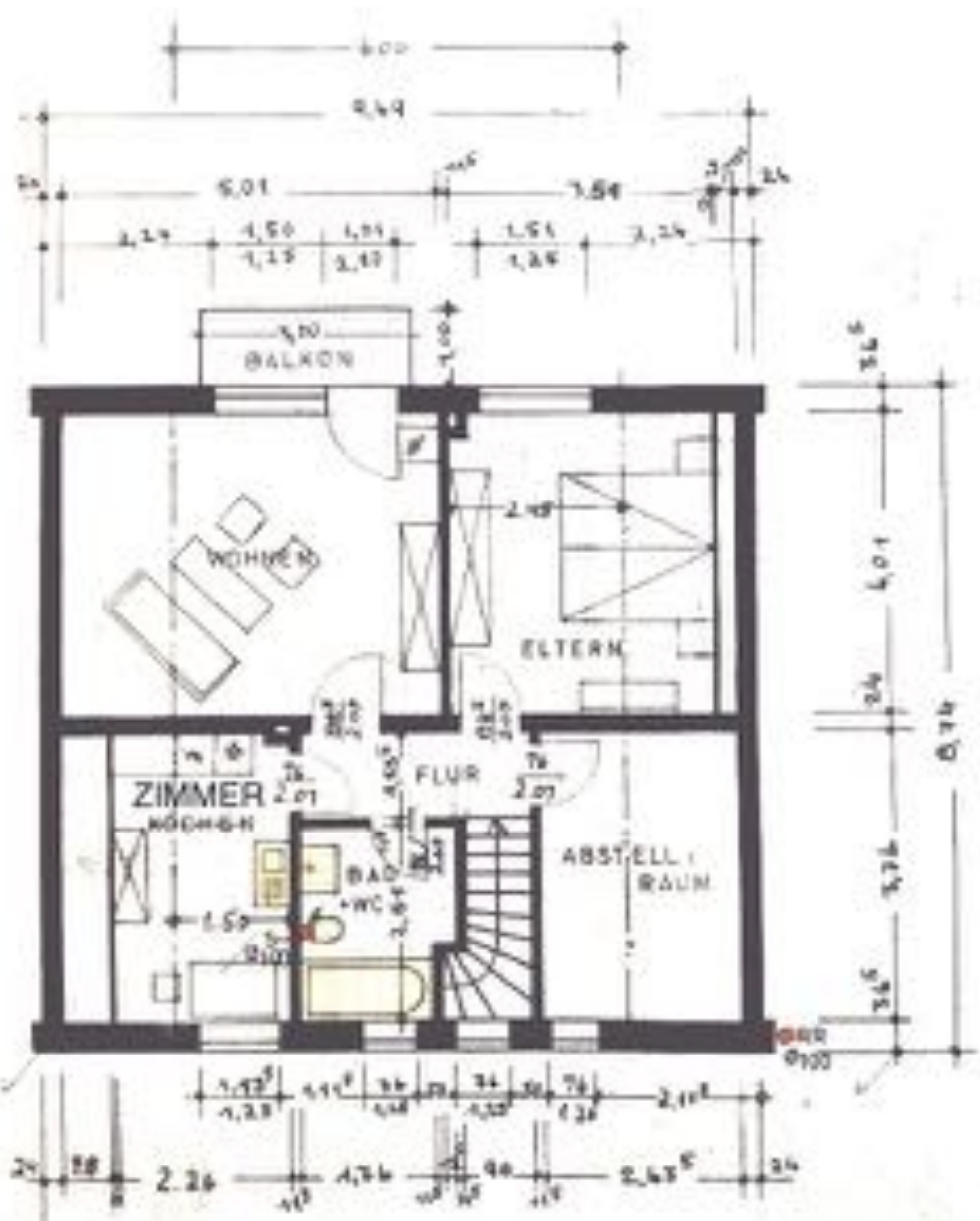
OBERGESCHOSS
