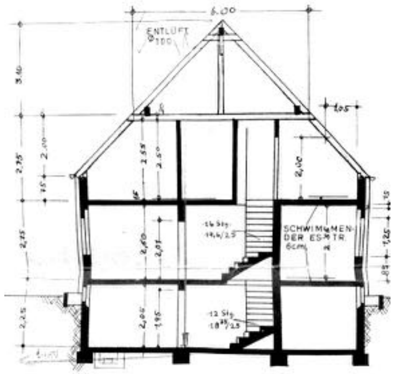
SCHNITT
